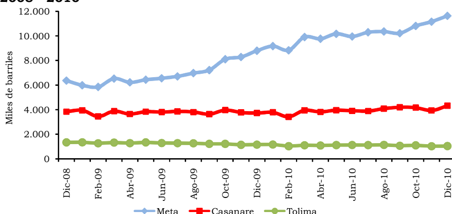
Gráfico 2.8.4.1. Casanare, Meta y Tolima. Producción mensual de petróleo 2008 - 2010
