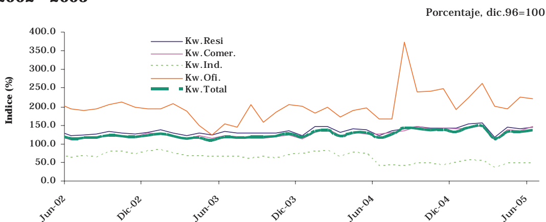
Gráfico 2.8.10.1 Caquetá. Índice de consumo de energía 2002 - 2005
